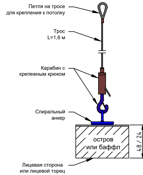
Схема крепления островов и баффов
