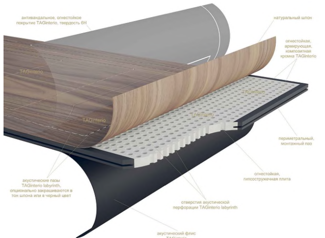
Панель TAGinterio перфорация Labyrinth
